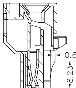
A-A SECTION
