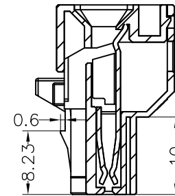
A-A SECTION
